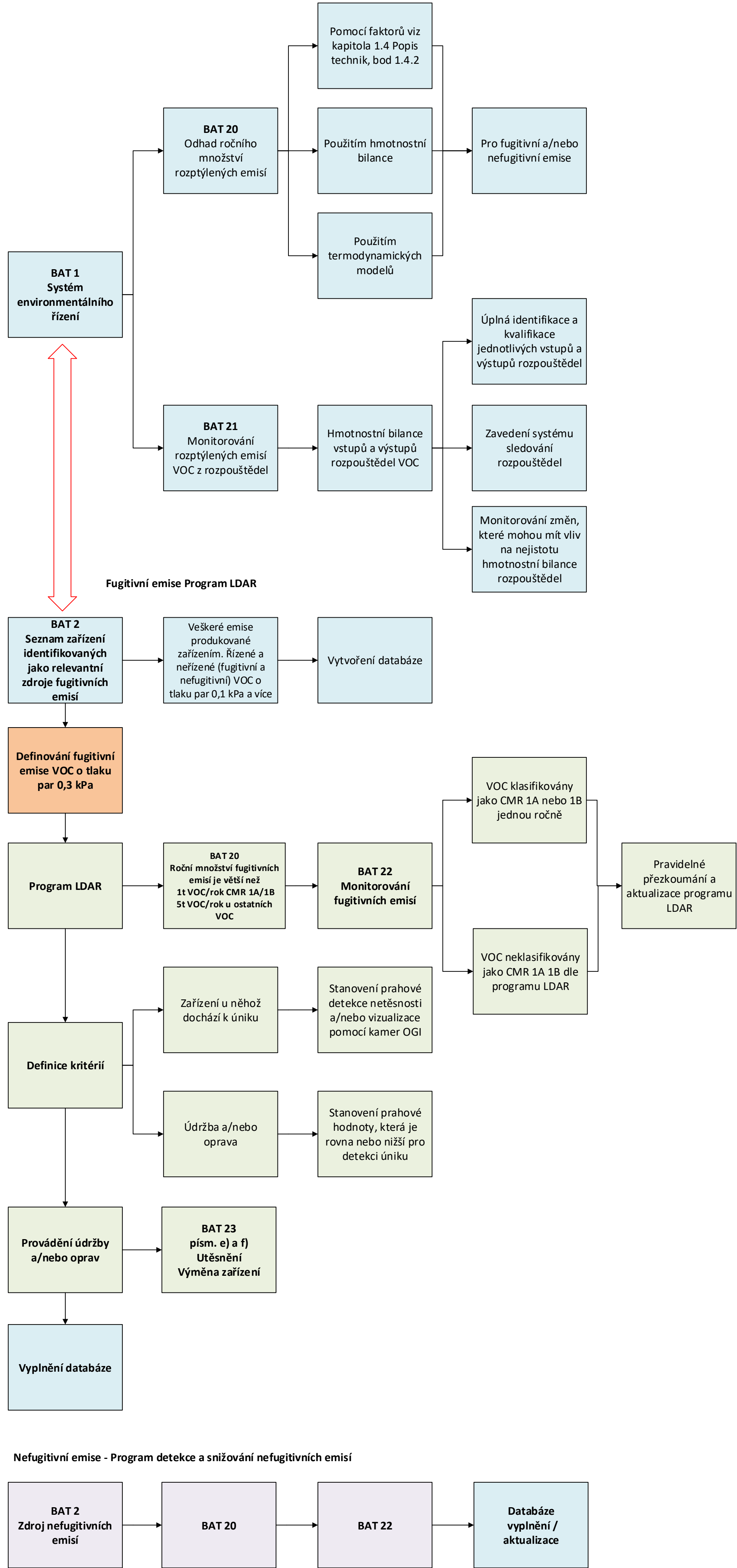
Příloha č. 3 Systém nakládání s rozptýlenými emisemi VOC
